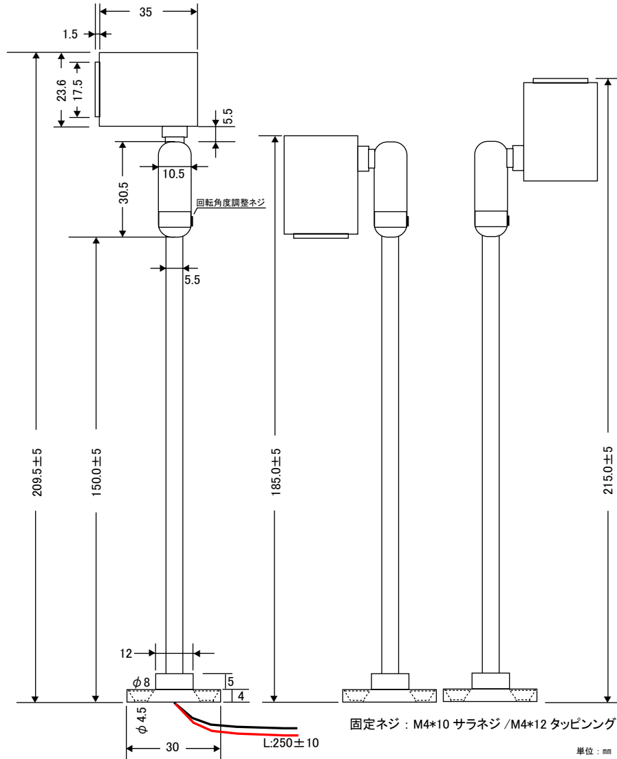
外形図: JCN-S-X001-CW-1W-75 / JCN-S-X001-WW-1W-75
